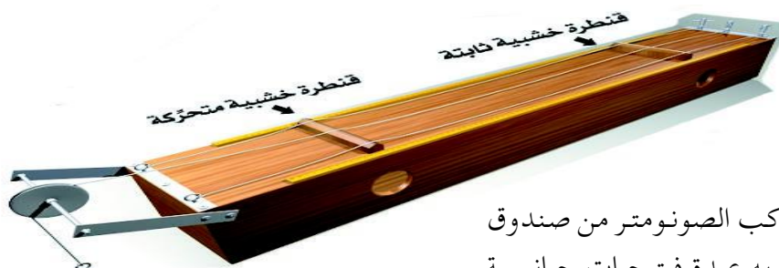
شكل (١٣) المصوات (الصونومتر)
