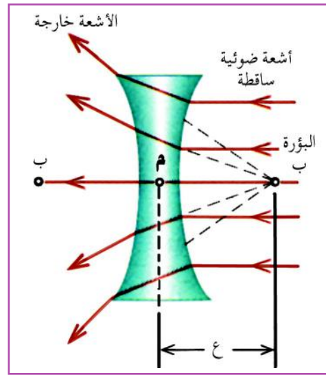
شكل (١٩) عدسة مقعرة (مفرقة).
